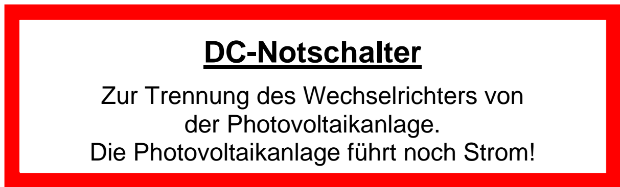
Abbildung 6: Kennzeichnung zur Trennung der DC/AC Geräte vom Hausnetz. Auf Seite der Photovoltaikanlage liegt der Strom noch an. Deutlich sichtbar in unmittelbarer Nähe des Schalters anzubringen.
